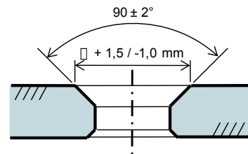
Bild 16: Senklochtoleranzen ( \varnothing = Durchmesser)
