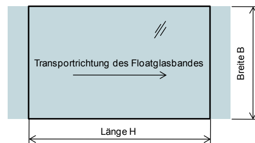
Bild 1: Länge H und Breite B von Bandmaßen und geteilten Bandmaßen
